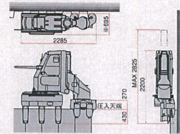
※はゼロ施工時寸法
